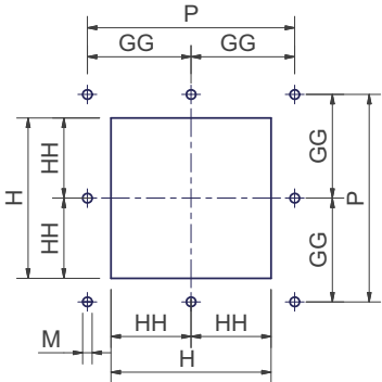
Foratura caldaia
