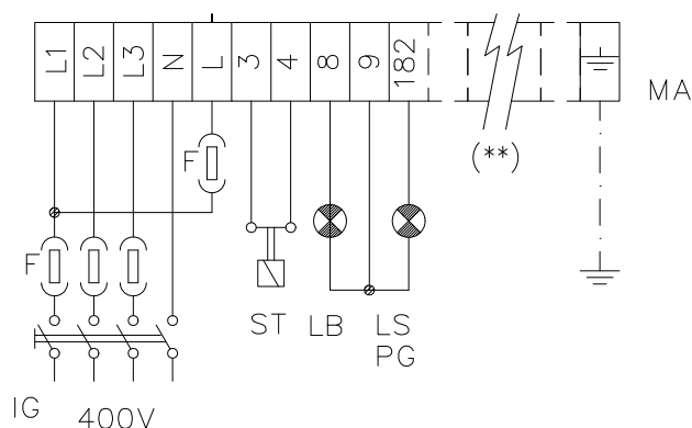
Fig. 3 - Bruciatori modulanti
