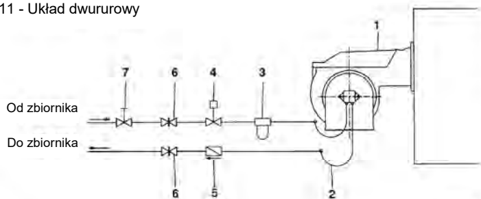
Rys. 11 - Układ dwururowy
