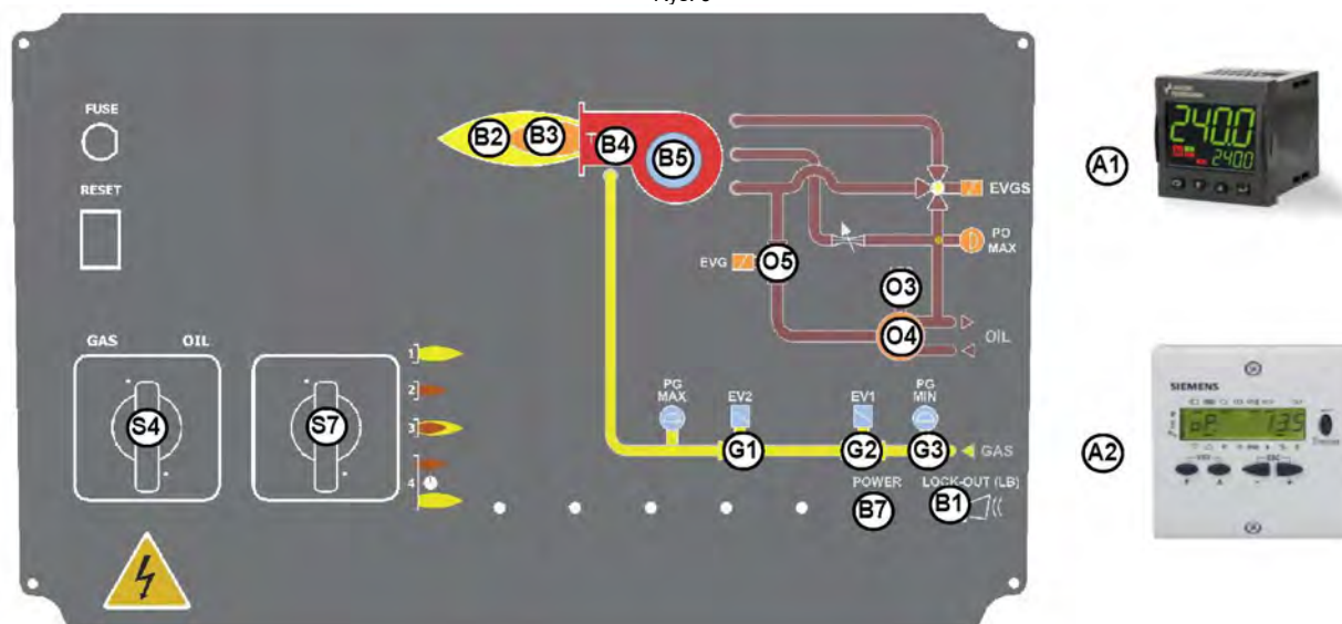
Rys. 10 - Przedni panel sterowania palnikiem
